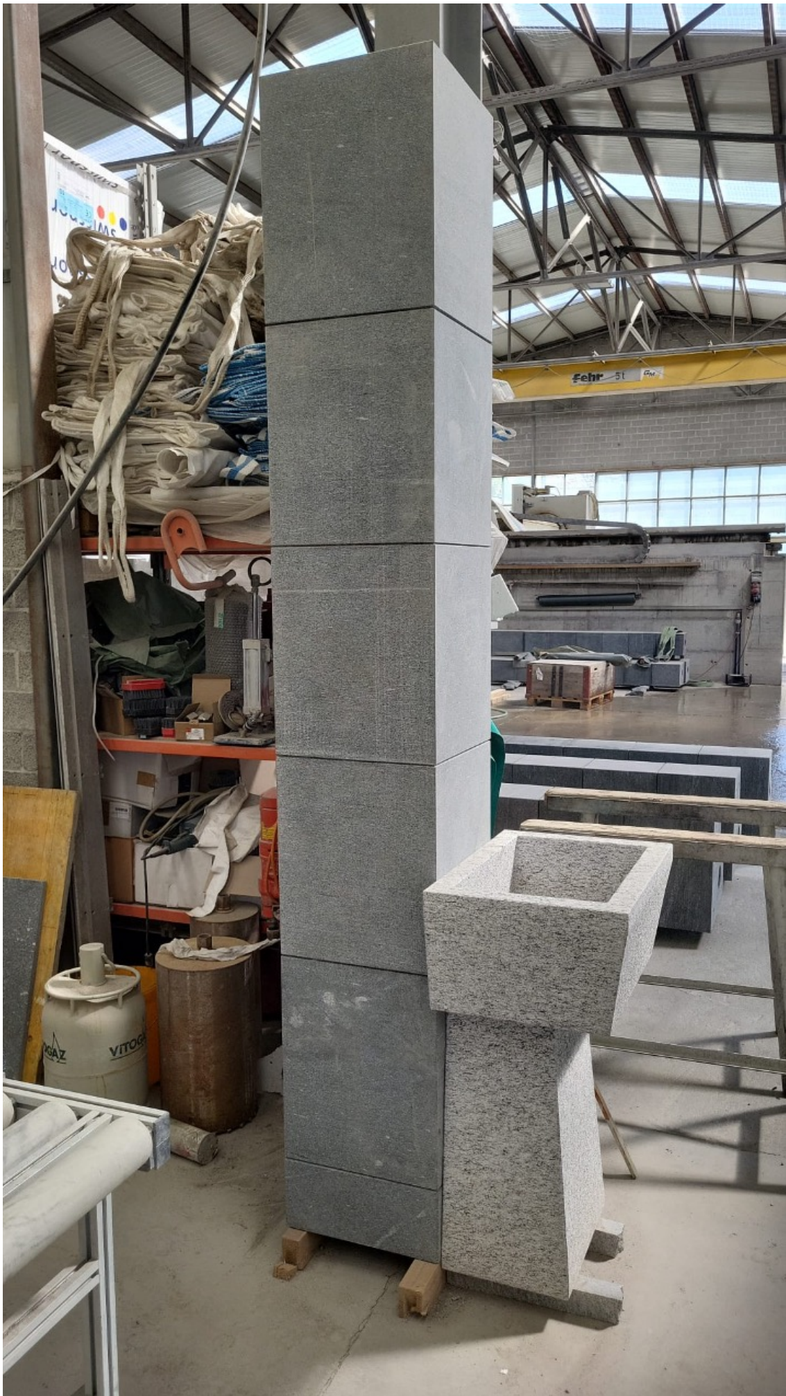
Tragende Steinstütze aus Bodio Nero mit den Massen 260cm x 40cm x 40cm und einem Gewicht von rund 1'100 Kg
