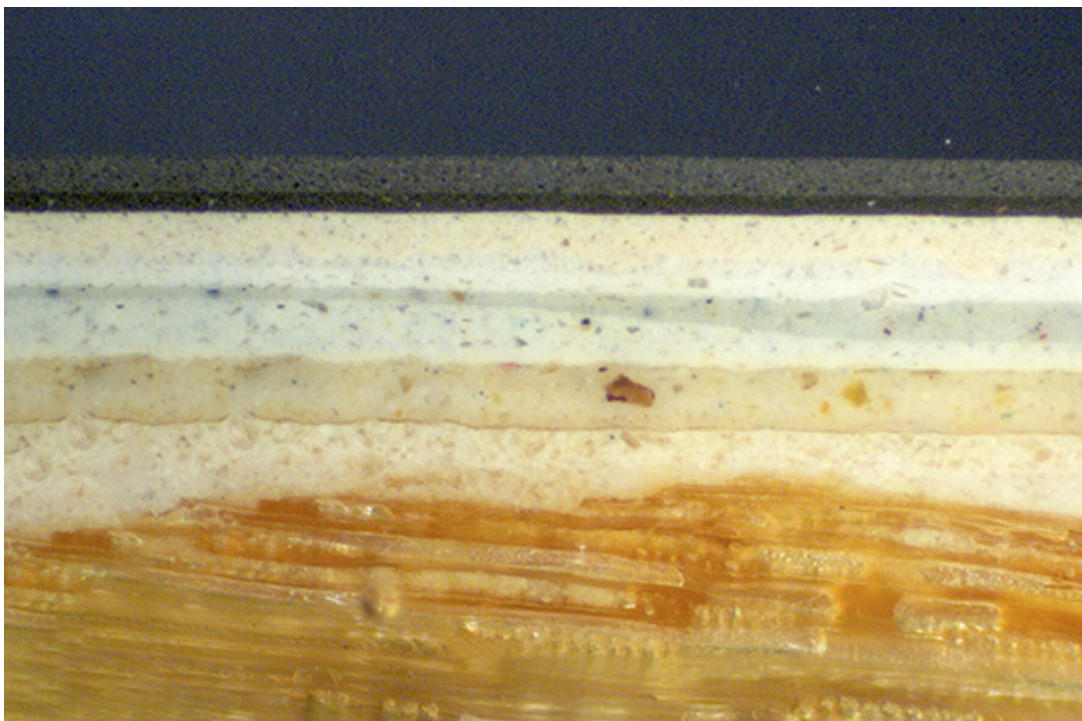
Schichtaufbau unter dem Mikroskop, Farb- und Anstrichanalyse Bild: Max Schweizer AG
