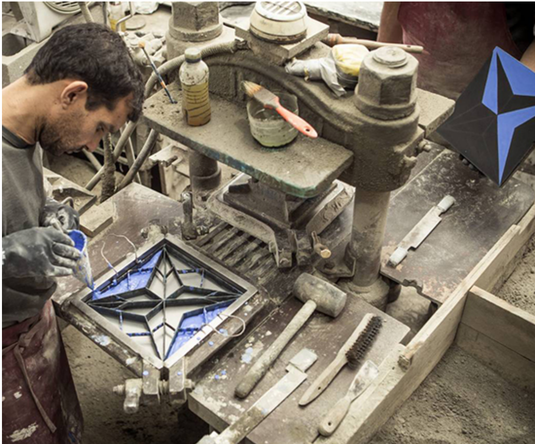
Herstellung der Zementfliesen
