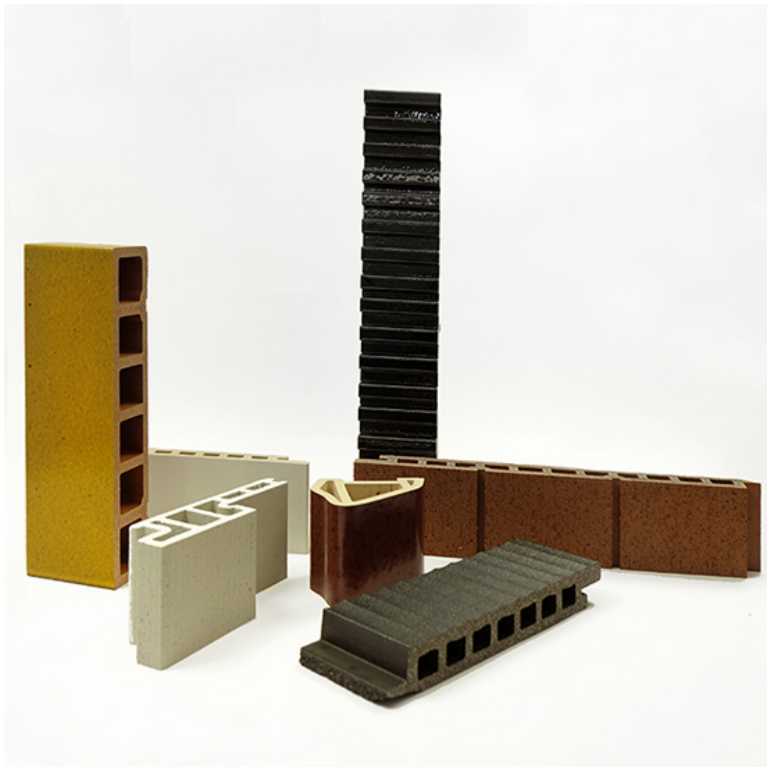
Stranggepresste Terra Cotta Formteile in der SBCZ Sammlung
